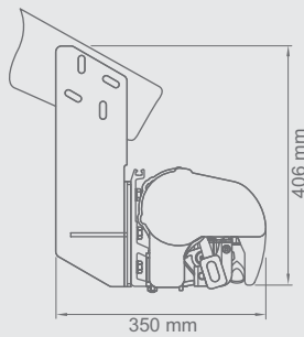
Stiprina pie spārēm Roof rafter installation Монтаж к кровли
