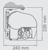
Stiprina pie griestiem Ceiling installation Потолочная установка
